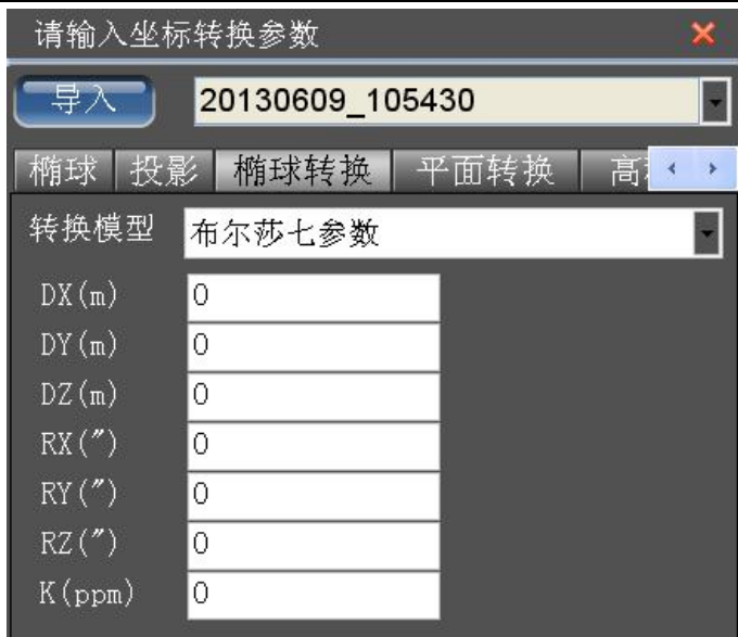
图 7-8 七参数
