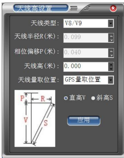
图 8-4 天线高计算
