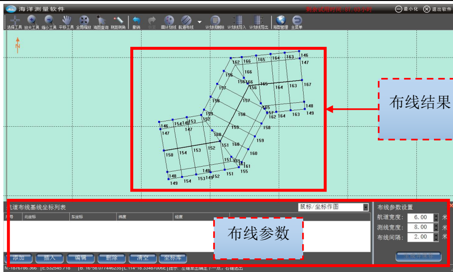
图 10-9 计划线布线
