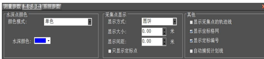
图 13- 14 显示参数
