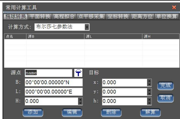
图 19-2 添加坐标点
