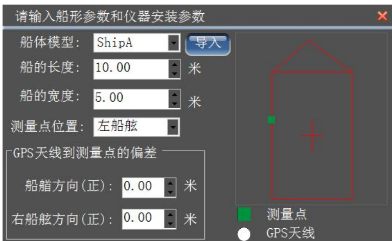
图 9-1 船形设计
