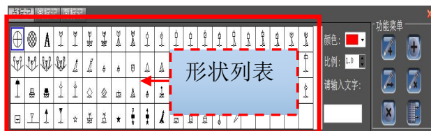
图 13-3 点标记
