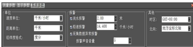
图 13-18 系统参数
