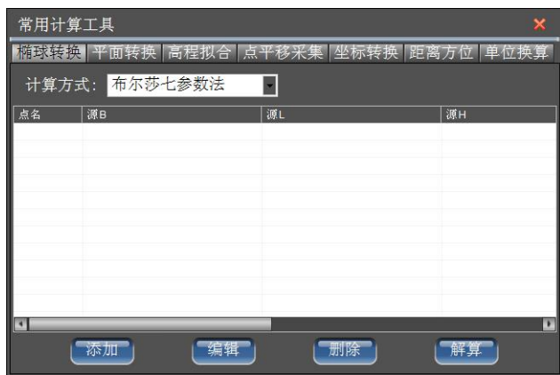
图 19-1 实用工具
