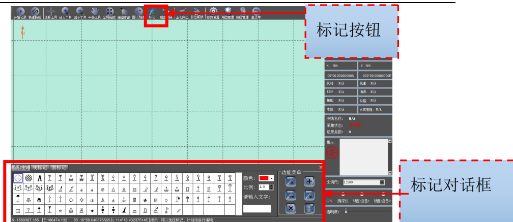
图 13-2 标记
