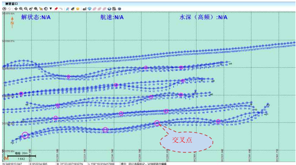
图 15-4 交叉点示意图
