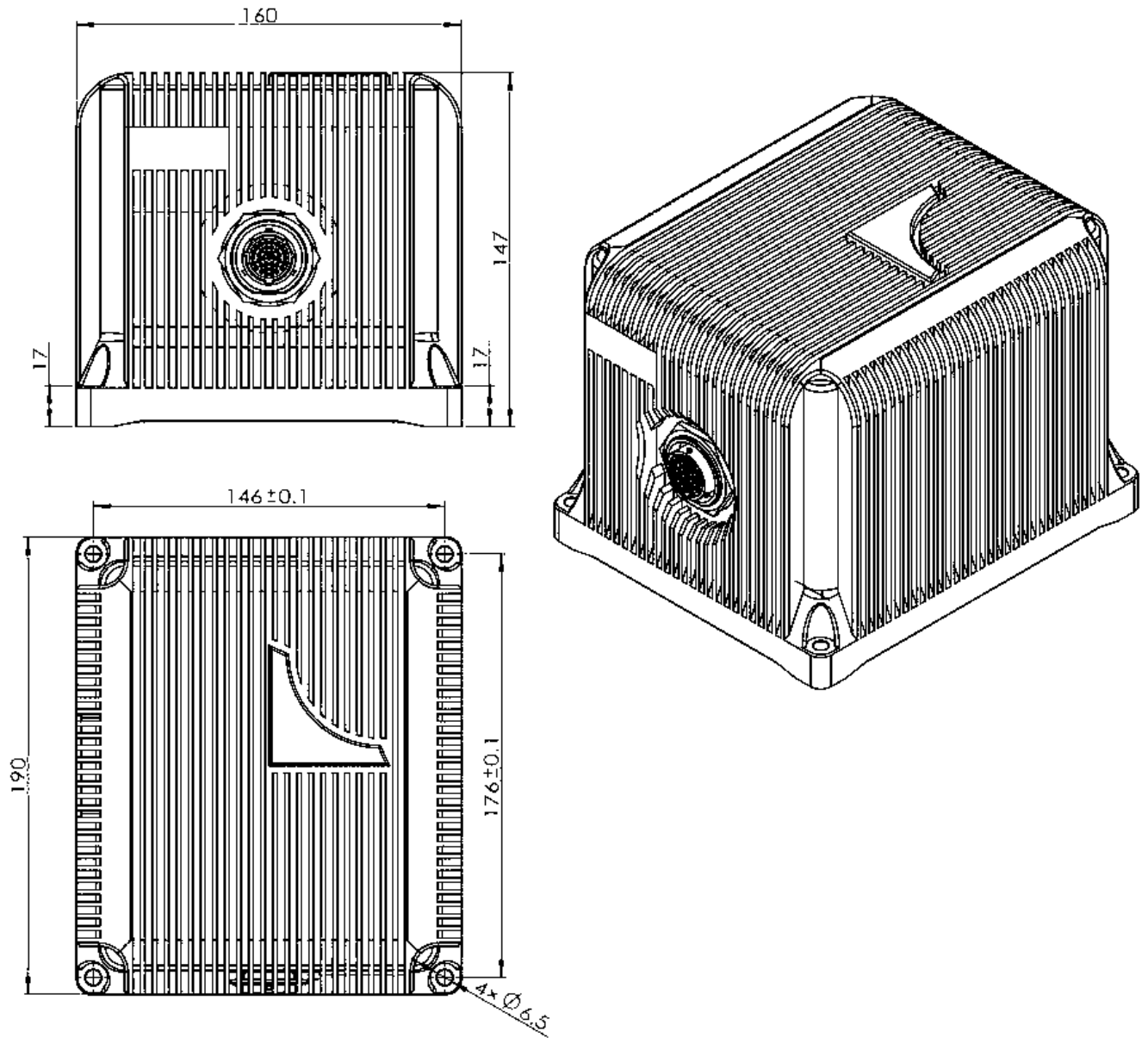
图 7.1 IMU 结构图
