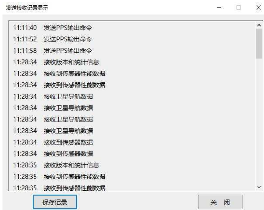
图 5.17 消息记录
