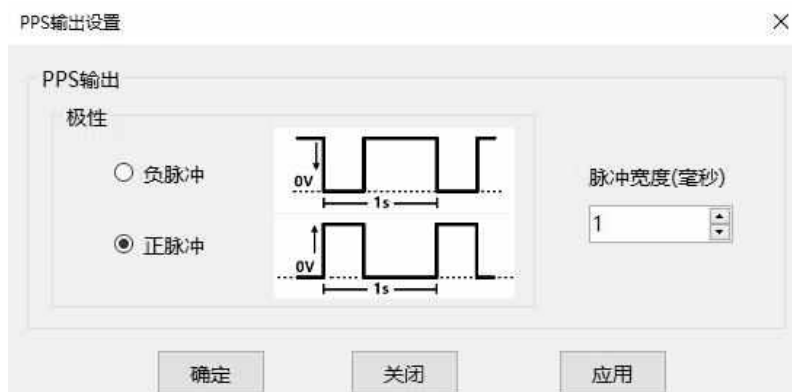
图 5.14 PPS 输出设置界面
