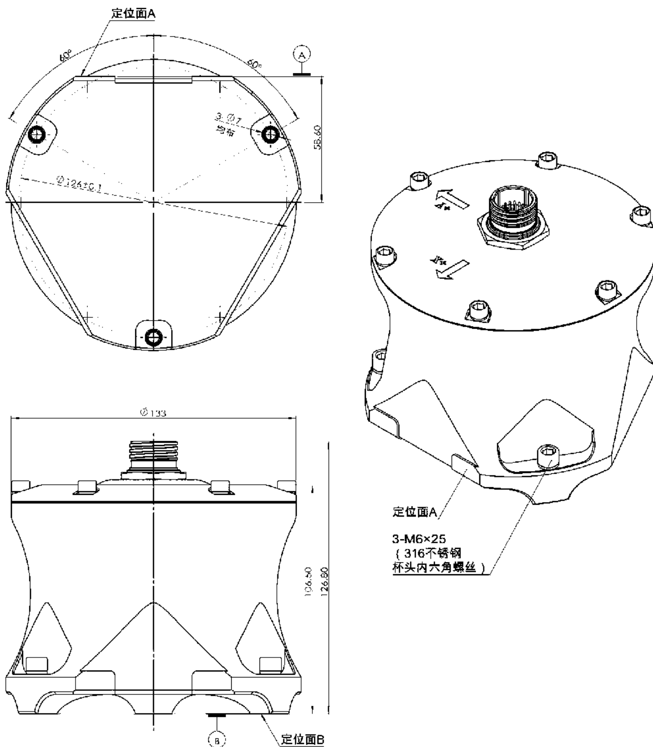
图 7.1 IMU 结构图
